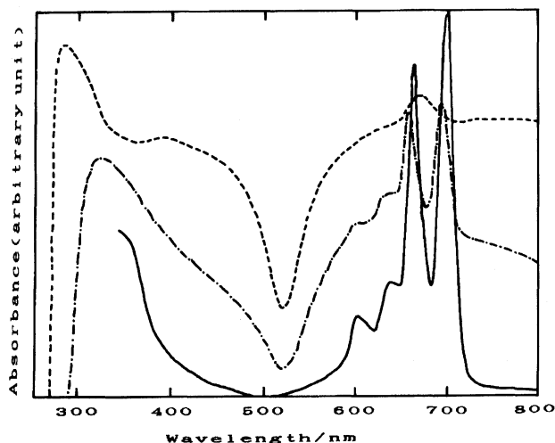
Fig. 8. Absorption spectra of H 2 pc in 1-Cl-naphthlene (—), HMPA (---), and DMSO (-.-).
